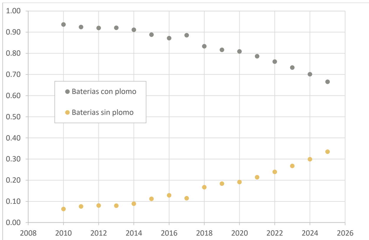
Figura 9-8 Participación histórica (2010-2019) y proyectada (2020-2025) según tipo de batería estacionaria,
